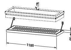
# 6443 ↔ 1180 mm, ↗ 440 mm
