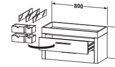
# 9267 ↔ 800 mm, ↗ 360 mm
