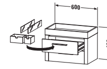
# 9266 ↔ 600 mm, ↗ 360 mm
