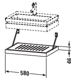
# 6441 ↔ 580 mm, ↗ 400 mm → # 6406
