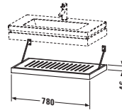
# 6442 ↔ 780 mm, ↗ 440 mm → # 6407
