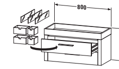
# 9267 ↔ 800 mm, ↗ 360 mm
