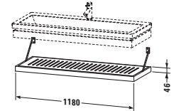
# 6443 ↔ 1180 mm, ↗ 440 mm → # 6408
