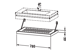
# 6442 ↔ 780 mm, ↗ 440 mm
