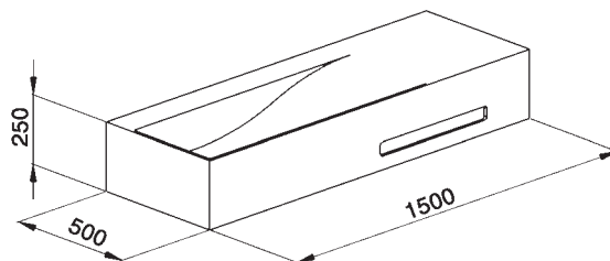
GA 00051 0 Lavabo 150x50 Wash-basin 150x50 Lavabo 150x50 Waschbecken 150x50 Lavabo 150x50
