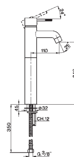
LS 00254 O Monocomando lavabo Single lever wash-basin mixer Mitigeur lavabo Einhand-Waschtischbatte Monomando lavabo
