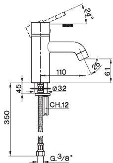
LS 00054 O Monocomando lavabo Single lever wash-basin mixer Mitigeur lavabo Einhand-Waschtischbatte Monomando lavabo
