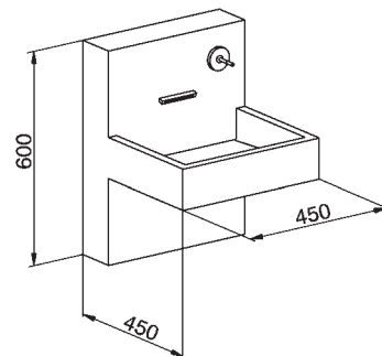
GA 00049 0 Lavabo 45x45 Wash-basin 45x45 Lavabo 45x45 Waschbecken 45x45 Lavabo 45x34
