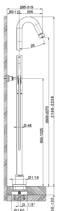
ST 00510 O Colonna doccia Shower column Colonne douche Standbrause Columna de ducha de suelo
