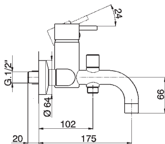
LM 00015 0 Monocomando vasca Single lever bath mixer Mitigeur bain/douche Einhand-Badebatte Monomando bañera
