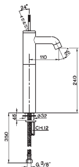
LS 00354 O Monocomando lavabo Single lever wash-basin mixer Mitigeur lavabo Einhand-Waschtischbatte Monomando lavabo
