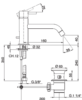
LM 00151 0 Monocomando lavabo Single lever wash-basin mixer Mitigeur lavabo Einhand-Waschtischbatte Monomando lavabo
