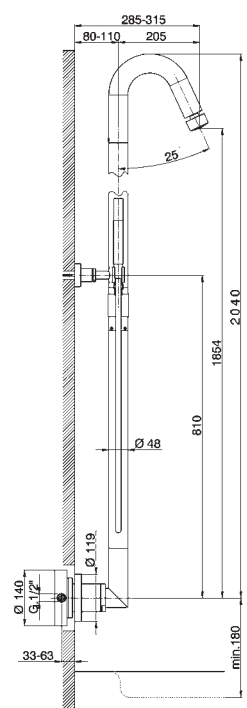
ST 00505 O Colonna doccia Shower column Colonne douche Standbrause Columna de ducha
