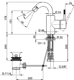
LS 00255 O Monocomando bidet Single lever bidet mixer Mitigeur bidet Einhand-Bidetbatterie Monomando bidé
