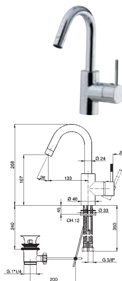
LS 00050 0 Monocomando lavabo Single lever wash-basin mixer Mitigeur lavabo Einhand-Waschtischbatterie Monomando lavabo
