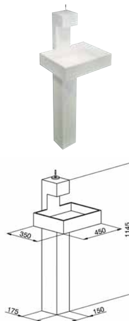
GA 00048 0 Lavabo a colonna 45x35 Wash-basin column 45x35 Colonne lavabo 45x35 Waschbecken in Säulenform 45x35 Lavabo de columna 45x35
