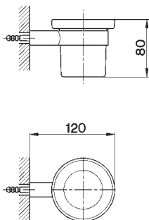
SY 09050 0 Porta bicchiere Glass holder Porte-verre Glashalter Portavasos
