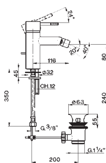
LS 00055 O Monocomando bidet Single lever bidet mixer Mitigeur bidet Einhand-Bidetbatte Monomando bidé
