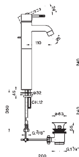
LS 00052 O Monocomando lavabo Single lever wash-basin mixer Mitigeur lavabo Einhand-Waschtischbatterie Monomando lavabo
