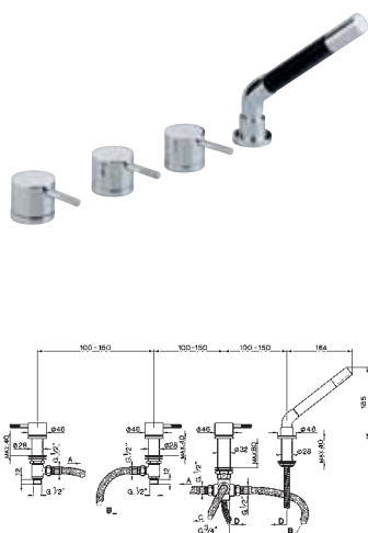
LS 00029 0 Batteria bordo vasca a 4 fori Deck-mounted 4-hole bath mixer Mélangeur B/D 4-trous sur gorge 4 Loch - Badebatterie Batería borde bañera de 4 agujeros
