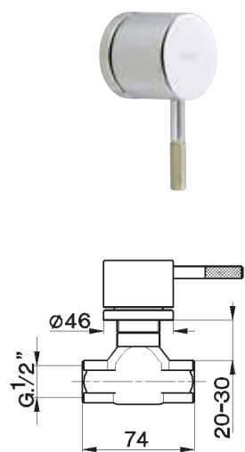
LS 00031 0 Rubinetto incasso Concealed valve Robinet à encastrer UP-Ventil Grifo para empotrar
