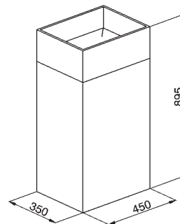
GA 00055 0 Lavabo a colonna 45x35 H. 90 Wash-basin column 45x35 H. 90 Colonne lavabo 45x35 H. 90 Waschbecken in Säulenform 45x35 H. 90 Lavabo de columna 45x35 H.90
