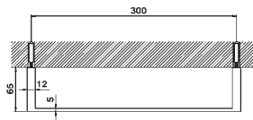
QU 09010 0 Portasalviette Towel holder Porte-serviettes Handtuchhalter Toallero
