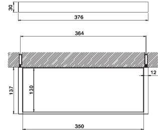
QU 09044 0 Porta mensola Shelf's holder Appui pour console KonsoleSpagnolo Portarepisa
