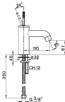
LS 00154 O Monocomando lavabo Single lever wash-basin mixer Mitigeur lavabo Einhand-Waschtischbatte Monomando lavabo
