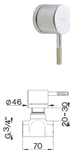
LS 00030 0 Rubinetto incasso Concealed valve Robinet à encastrer UP-Ventil Grifo para empotrar 3/4"
