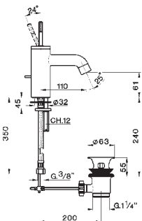
LS 00151 O Monocomando lavabo Single lever wash-basin mixer Mitigeur lavabo Einhand-Waschtischbatterie Monomando lavabo
