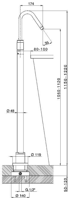
ST 00451 0 Colonna lavabo Wash-basin column Colonne lavabo Standwaschtisch Columna de lavabo
