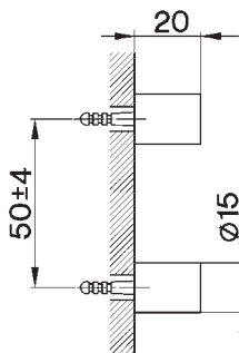
SY 09066 0 Set di installazione porta scopino a muro Set de instalación para porta escobilla a pared Toilet brushed holder Juego de instalación portaescobilla de pared
