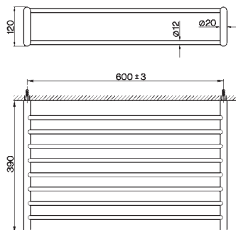
SY 09030 0 Griglia porta salviette Towel rack Étagère serviettes Handtuchablage Toallero de rejilla
