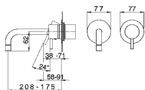
LM 00551 0 Parte esterna monocomando lavabo incasso Visible parts for single lever wash-basin concealed mixer Façade seule pour mitigeur lavabo encastré UP-Einhand-Waschtischbatterie - Fertigmontageset Parte exterior monomando lavabo para empotrar
