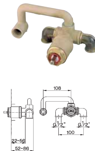
ZA 00651 0 Corpo monocomando lavabo incasso Concealed single lever wash-basin mixer Corps mitigeur lavabo encastré Einhand-UP-Waschtischbatterie Cuerpo monomando lavabo para empotrar
