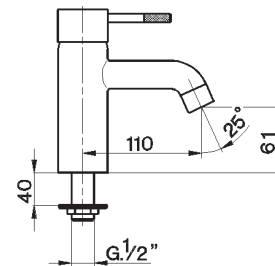
LS 00090 O Monoforo lavamani Pillar tap Robinet de comptoir Standventil Monobloc lavamanos
