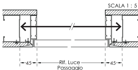
telaio a 4 lati
