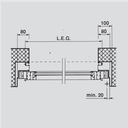
Sezione orizzontale
