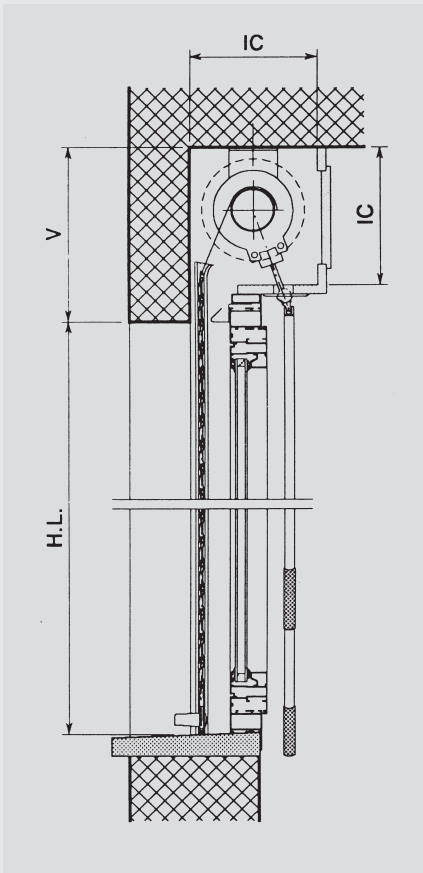
Sezione verticale
